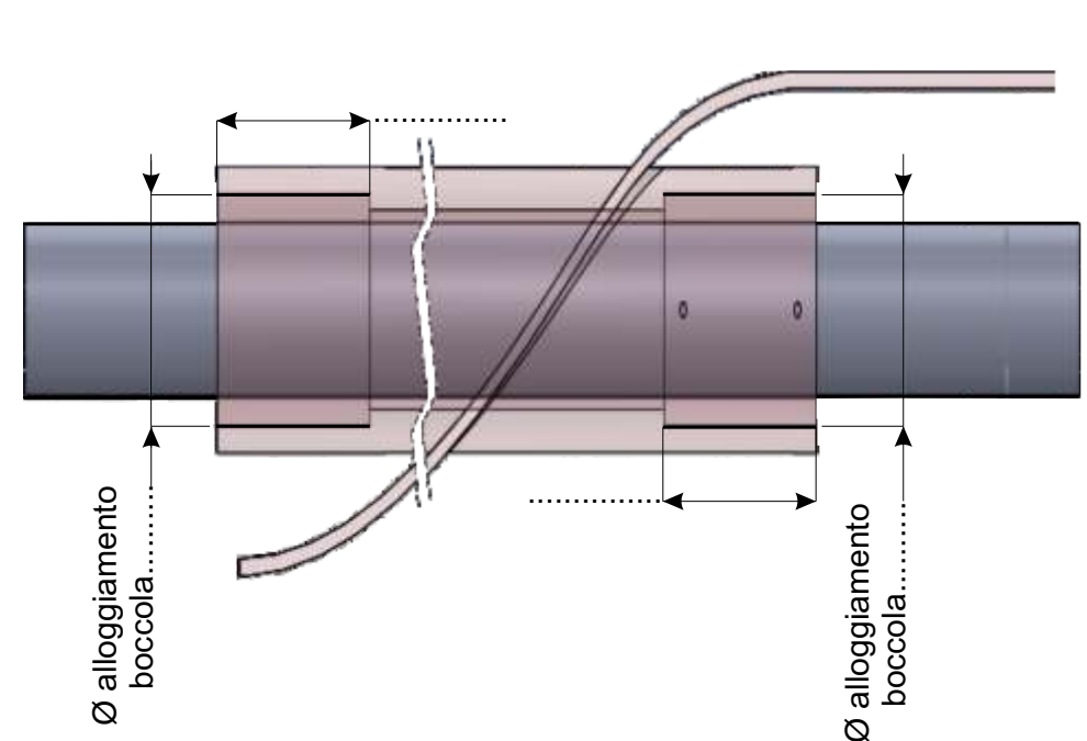
TUBO PASSASCAFO
